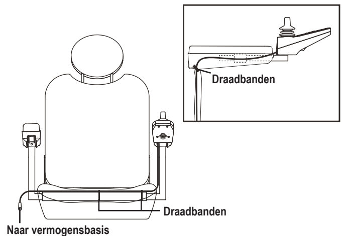
Figuur 8. Regelaar harness routing op een omtrekzitting
