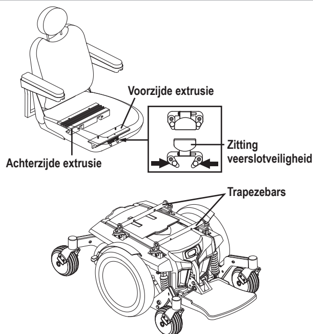
Figuur 6. Universeel montagesysteem en omtrekzittingseat
