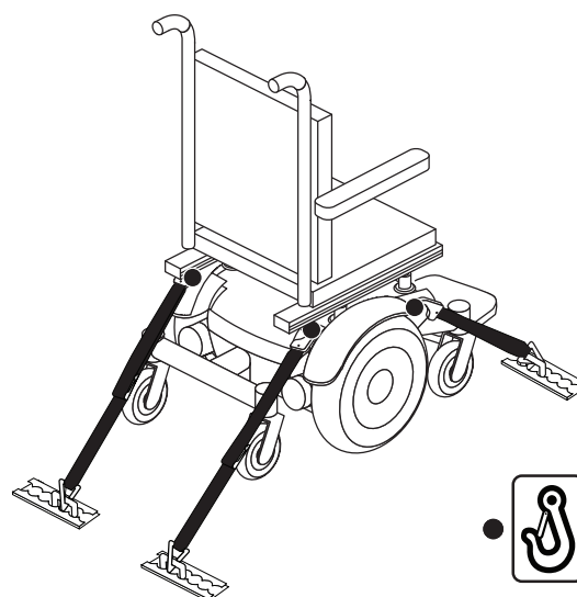
Figuur 12. Transitsysteem beveiligingssteunen
