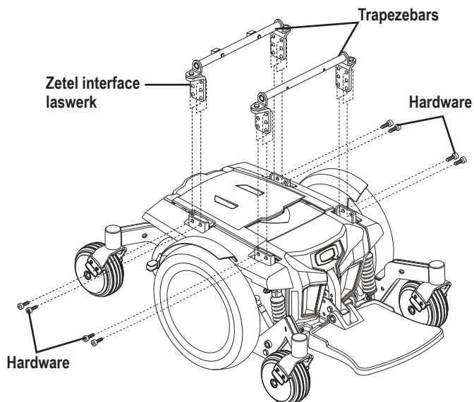
Figuur 14. Zittingshoogte/Hoekaanpassing
