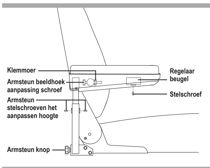
Figuur 16. Rugleuning/Armsteun instelling
