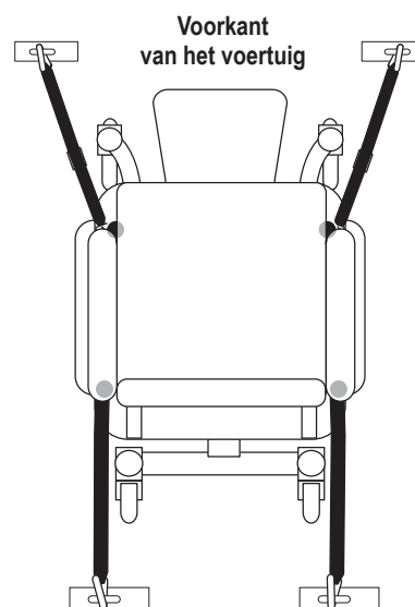
Figuur 13. Verzekeringbeugels voor leeg vervoerssysteem
