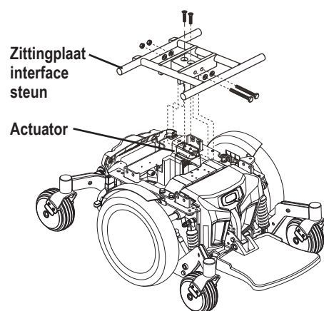
Figuur 11. Vermogen verhogende zitting actuator
