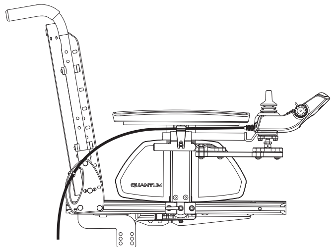
Figuur 9. Regelaar harness routing op een TB-Flex-zitting
