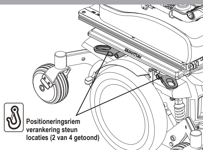
Figuur 12. Transitsysteem beveiligingssteunen
