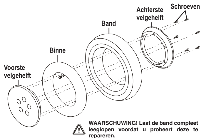
Figuur 23. Onderdelen drive-wiel
