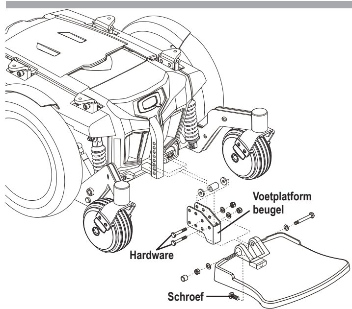
Figuur 17. Voet platform instelling
