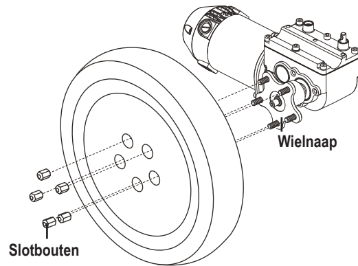
Figuur 22. Drive-wiel
