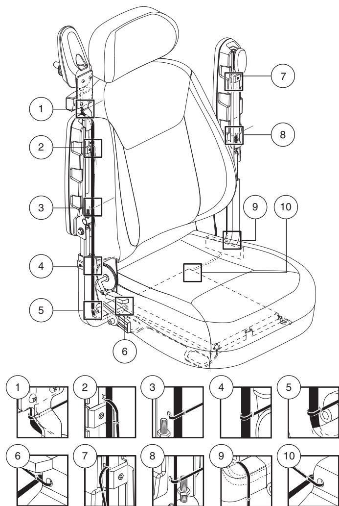
Figuur 10. Regelaar harnas routing op een zitting met iLevel
