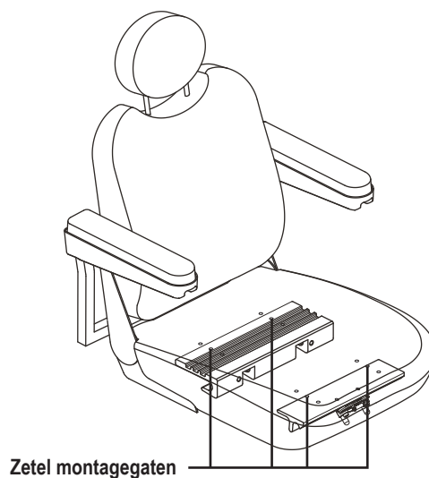
Figuur 15. Zetel positie instelling
